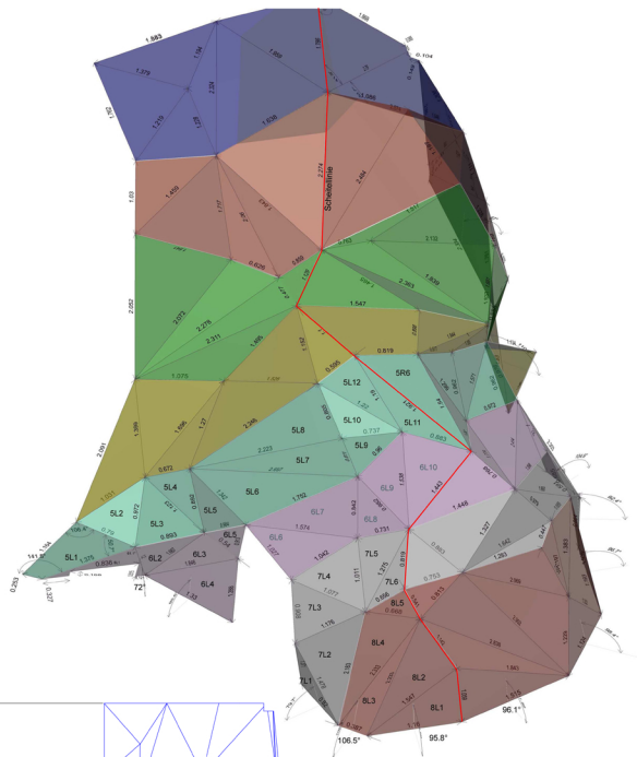
Isometrie linke Seite
