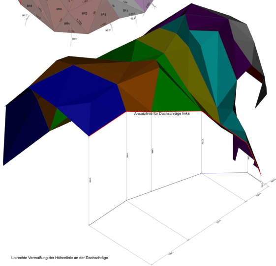
Lotrechte Vermaßung der Höhenlinie an der Dachschräge
